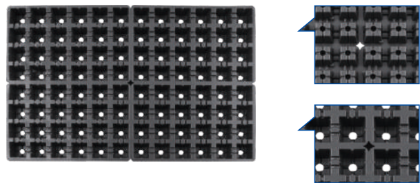
型号: TZSY-96 尺寸: 600 × 400 × 30mm
