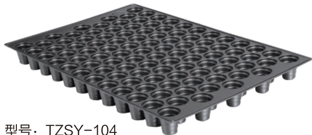
型号: TZSY-104 尺寸: 545 × 355 × 40mm
