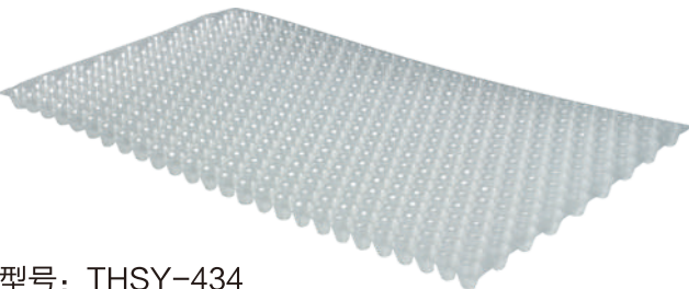
型号: THSY-434 尺寸: 600 × 330 × 16mm
